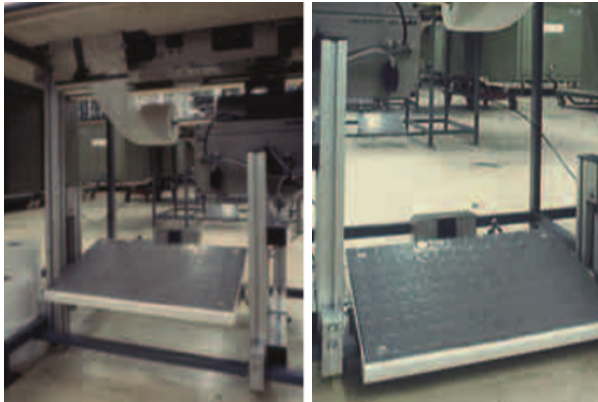
Figura 37. Pedal regulable en altura (Fuente: INSST, 2021).
