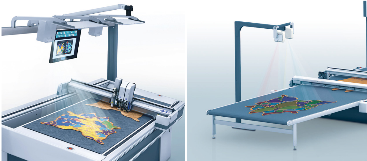
Figura 53. Sistema de proyección (Fuente: Zünd),
